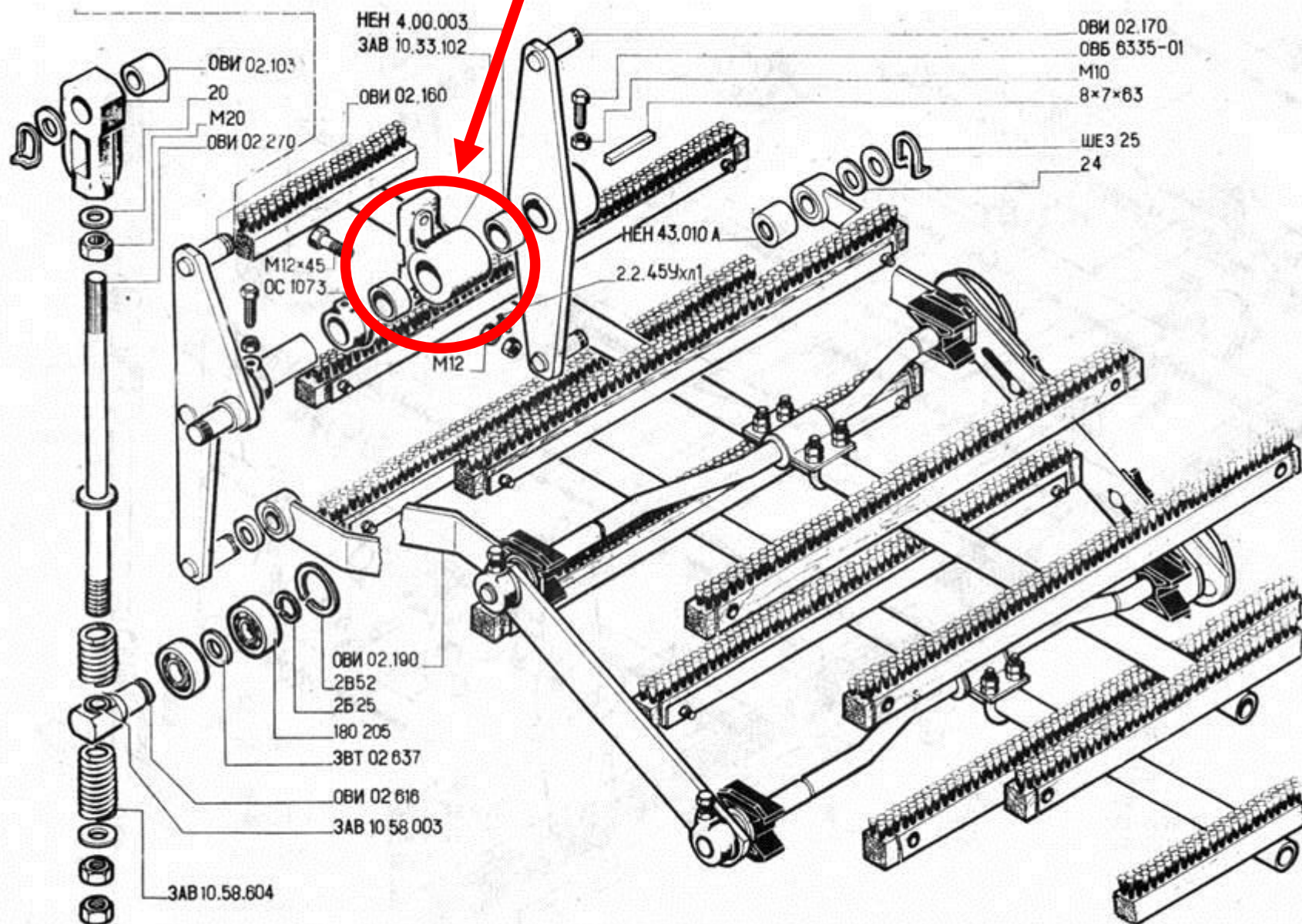
Рис. 12. Механизм очистки решет ОВИ 02.150.
